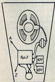
Rys. 3 Rozmieszczenie elementów odbiornika
